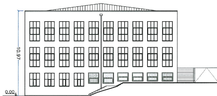
ALZADO NOROESTE
