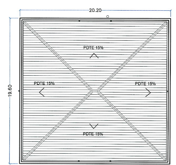
PLANTA CUBIERTA
