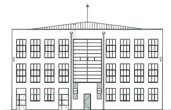
ALZADO NORESTE
