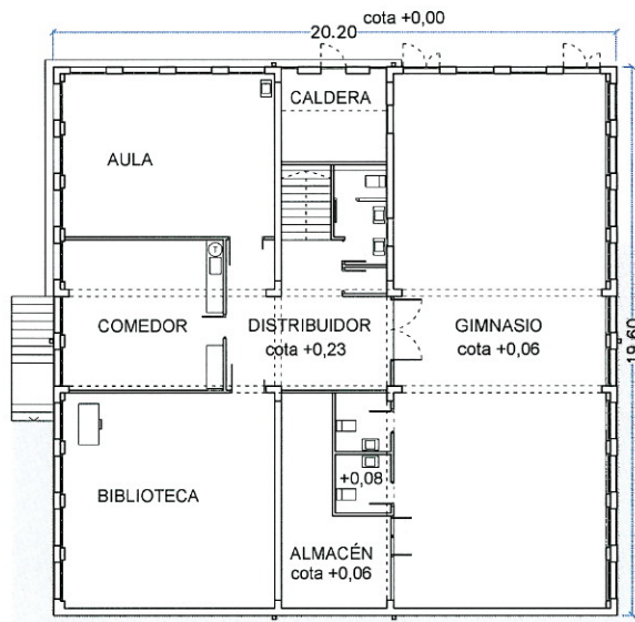
PLANTA SEMISÓTANO
