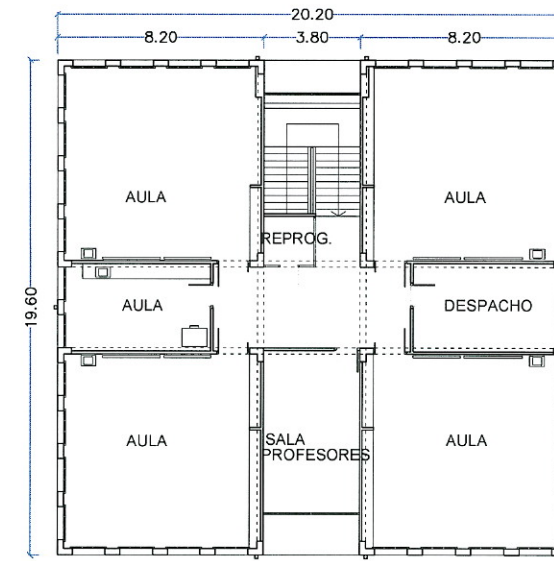
PLANTA PRIMERA
