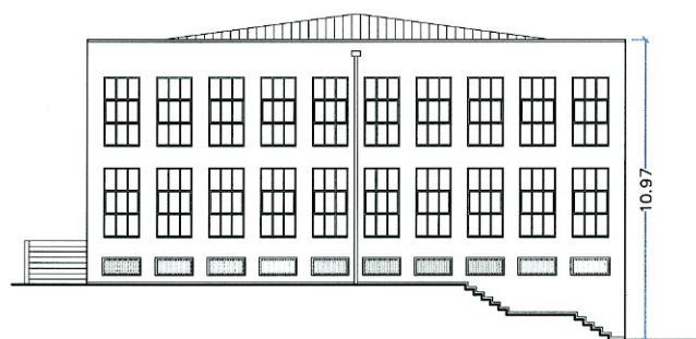
ALZADO SURESTE
