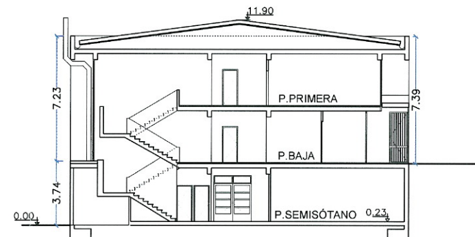
SECCIÓN B
