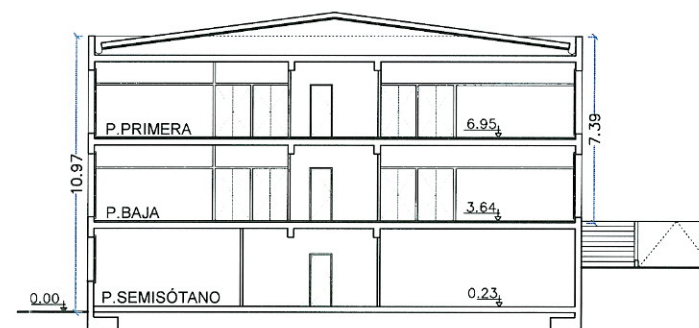
SECCIÓN A
