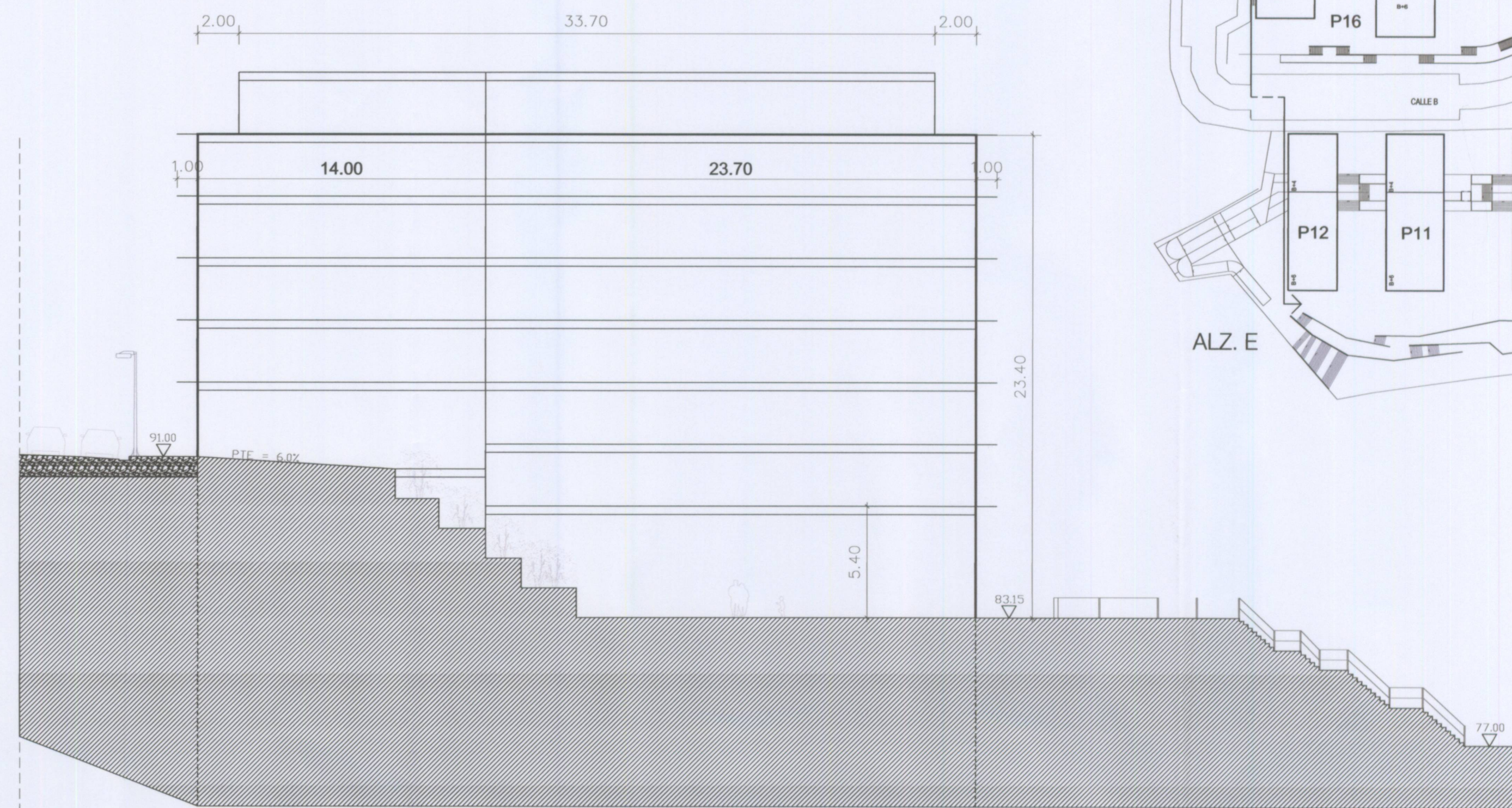
ALZADO E
