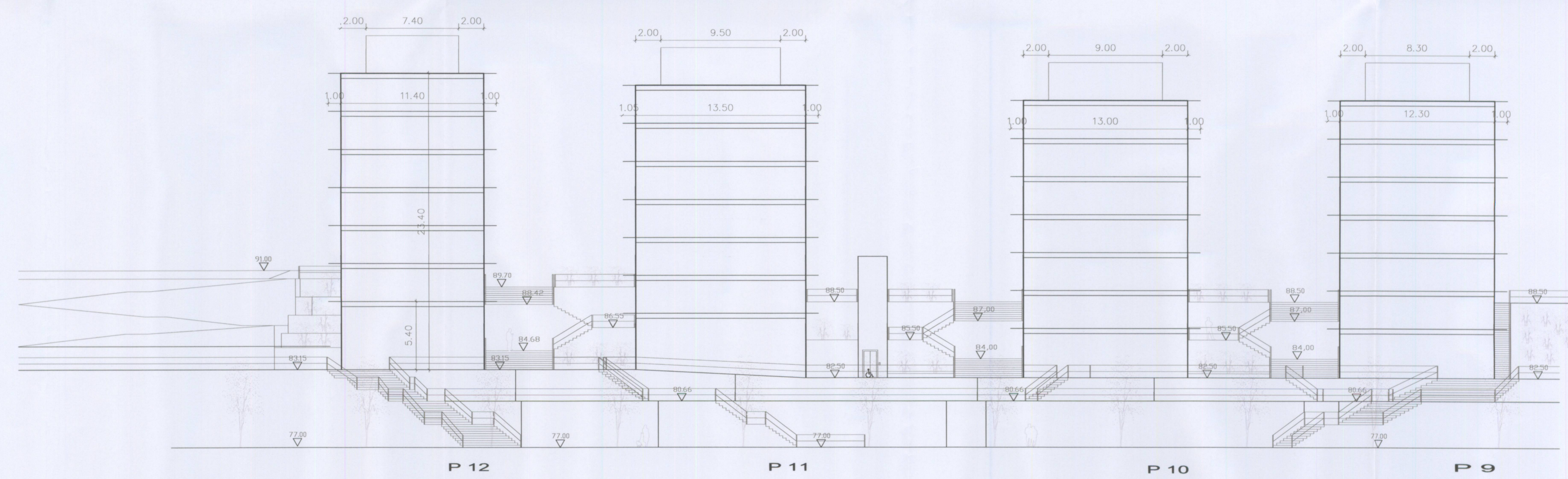
ALZADO D
