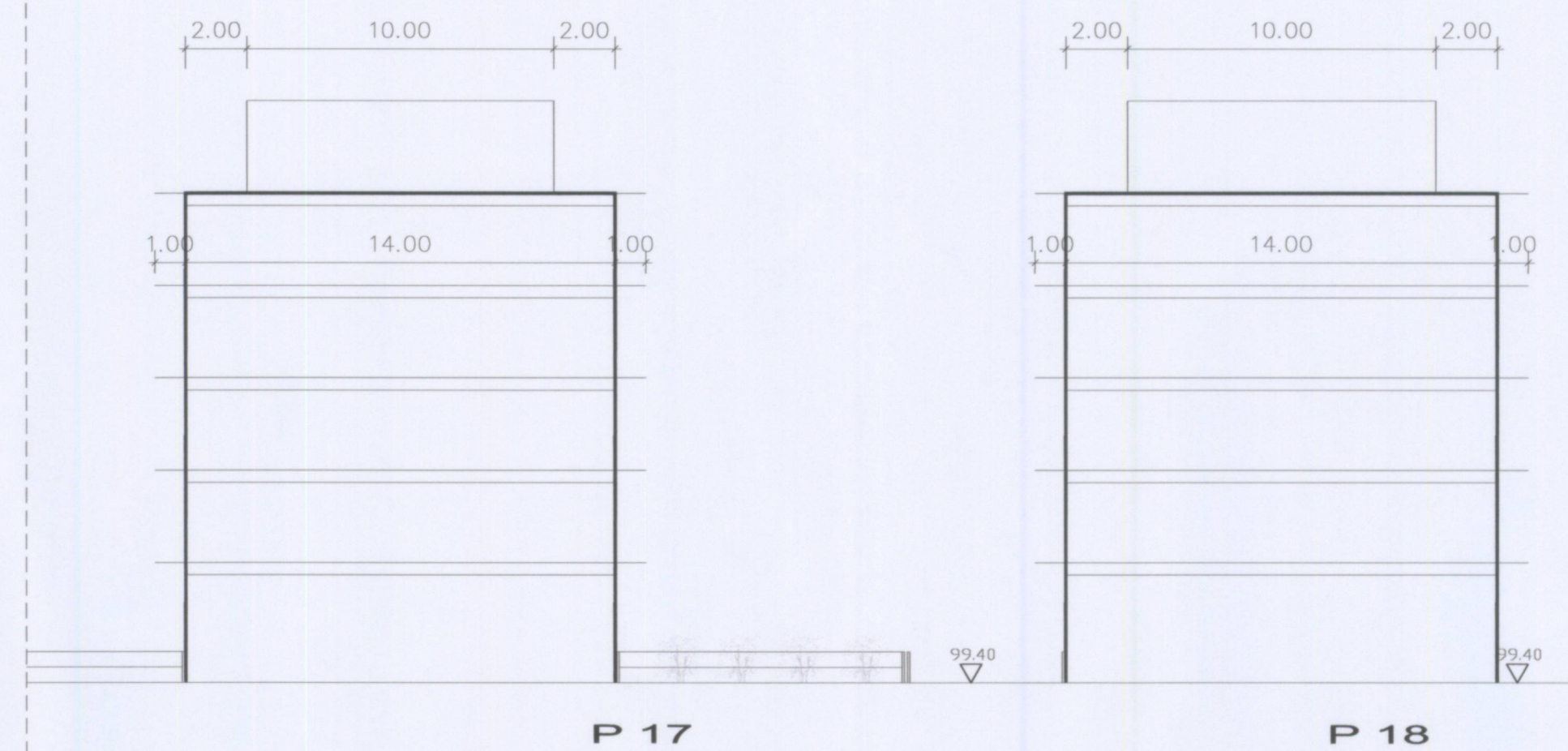
ALZADO A
