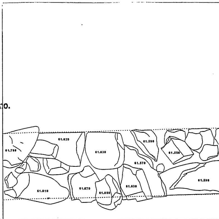
Perfil Sur
