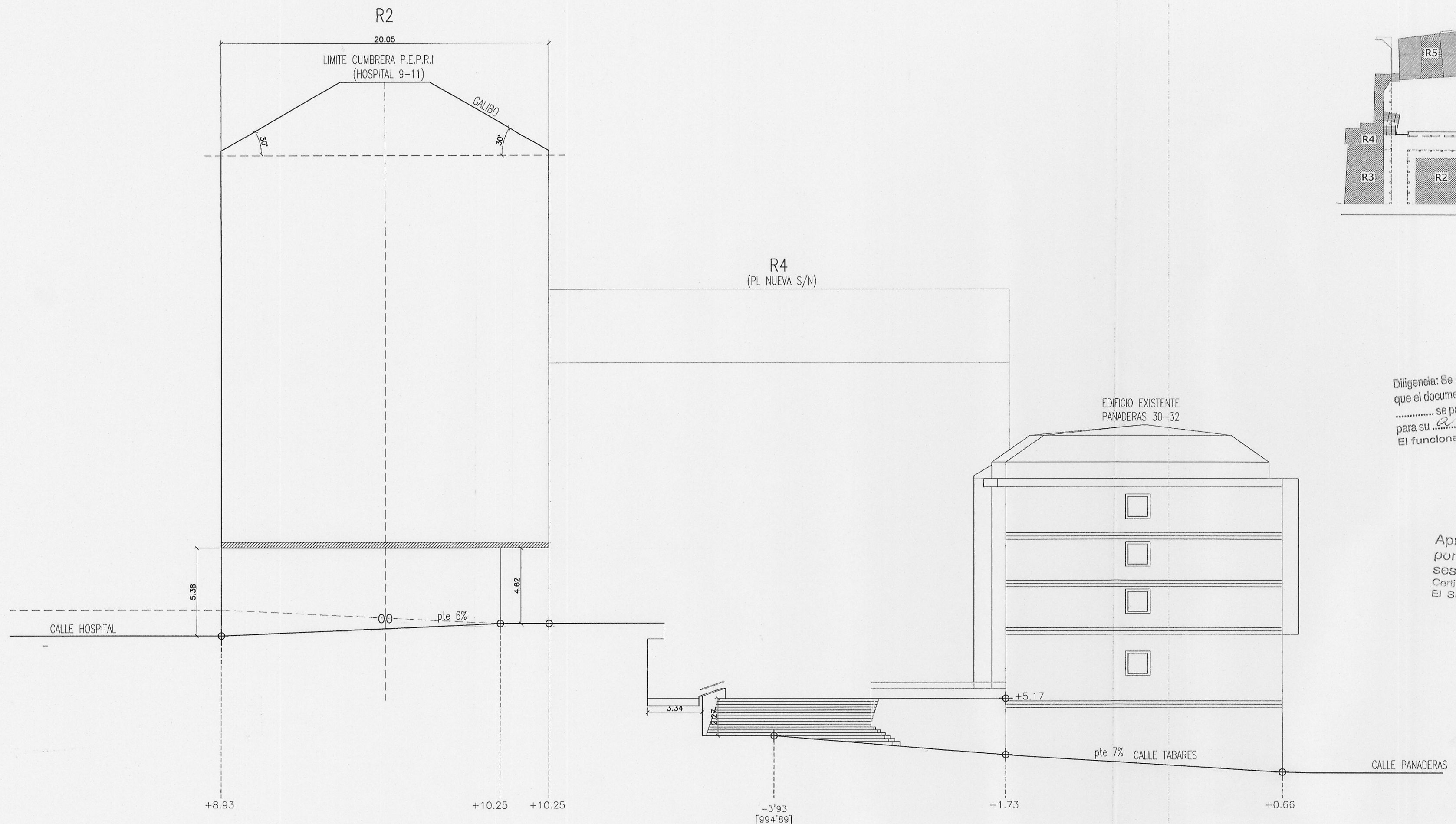
SECCION POR CALLE TABARES 2 ESCALA 1/200
