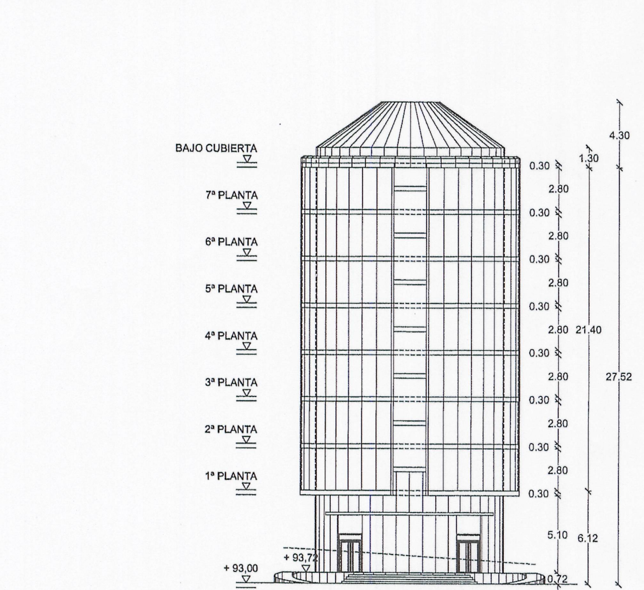
ALZADO TORRE
