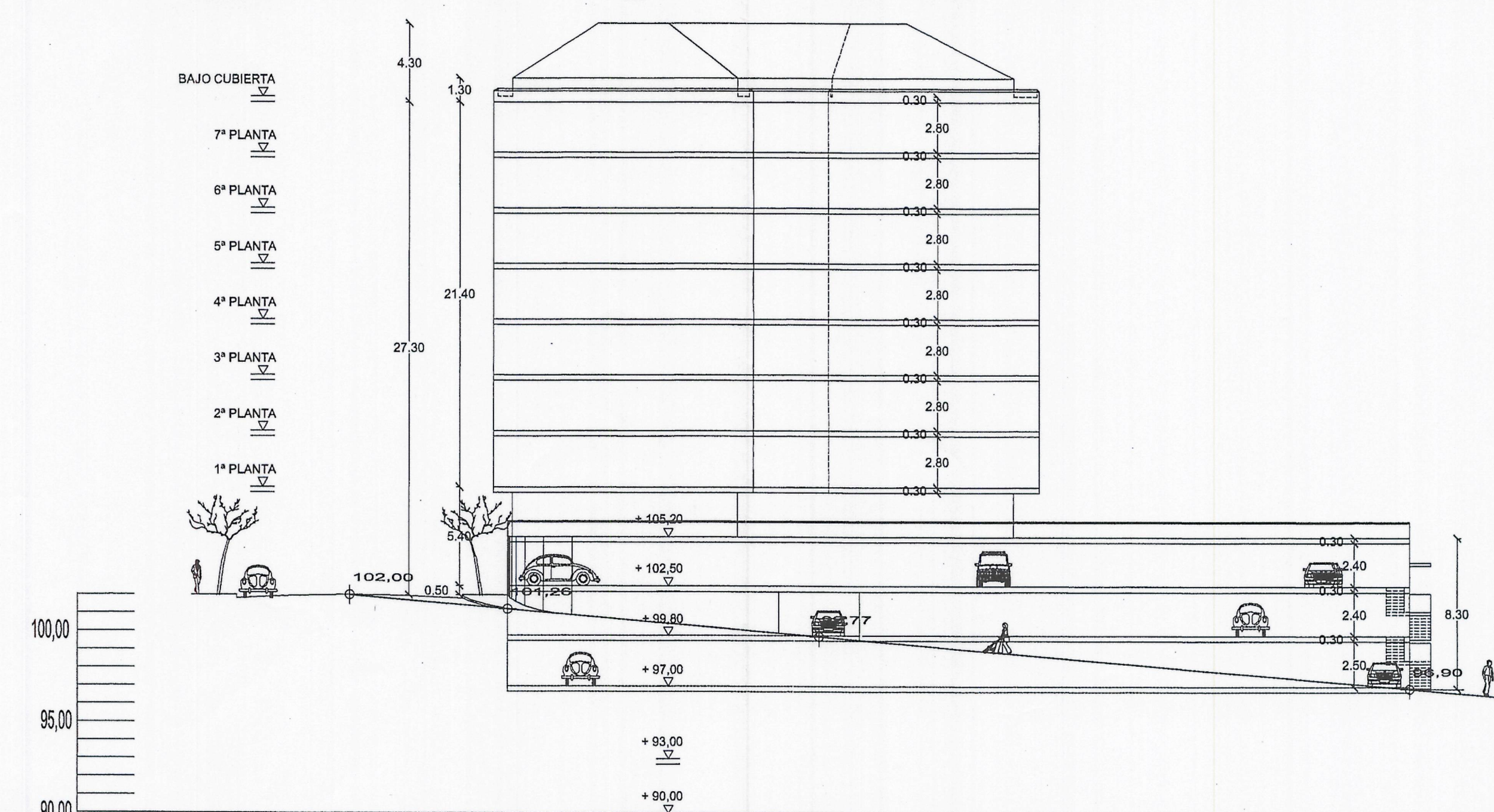
PERFIL OESTE
