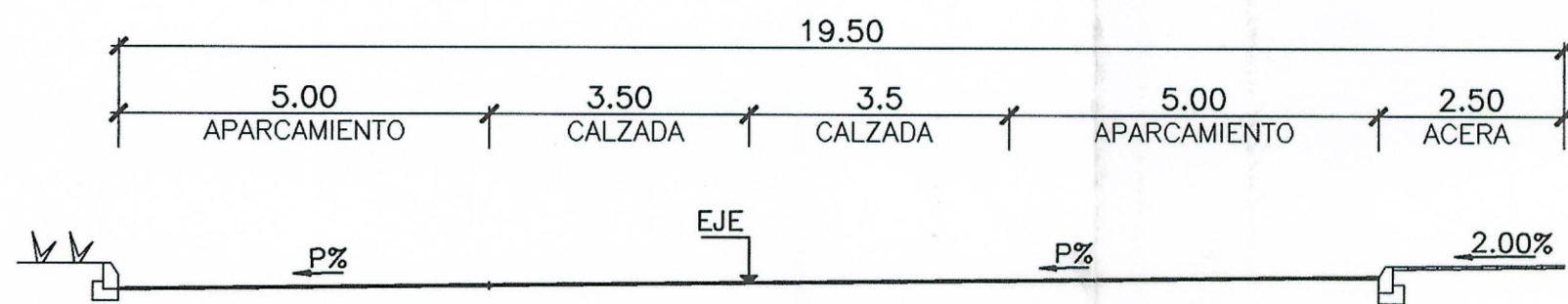
SECCION TIPO EJE BIDIRECCIONAL CON APARCAMIENTOS(VIA-2) ESCALA 1:100
