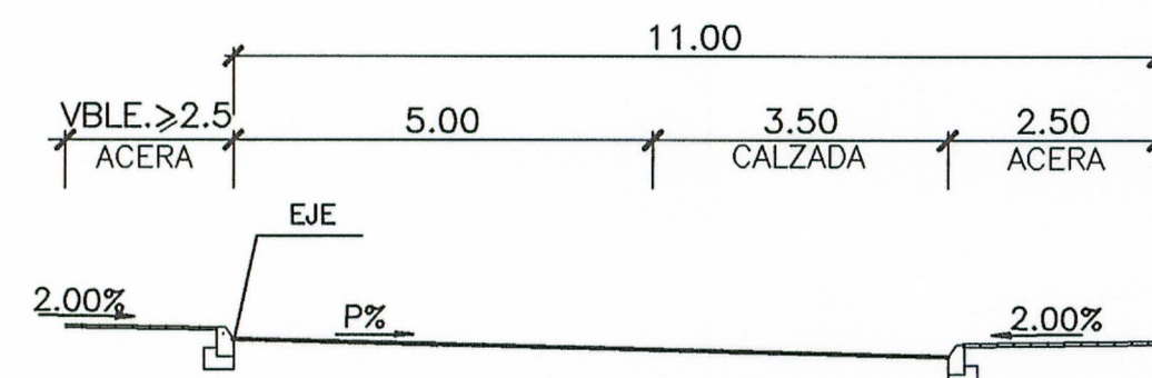
SECCION TIPO EJE UNIDIRECCIONAL CON APARCAMIENTOS(VIA-1) ESCALA 1:50
