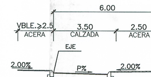
SECCION TIPO EJE UNIDIRECCIONAL(VIA-1) ESCALA 1:50
